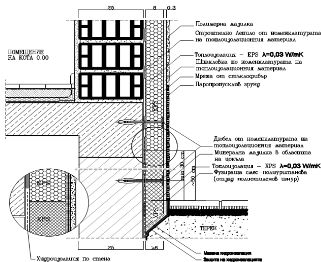
ДЕТАЙЛ "1" М 1:10
